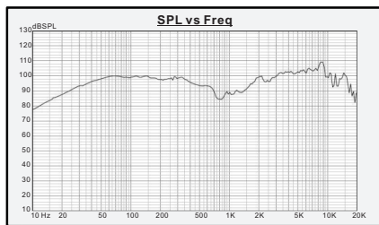
PH-1502频响曲线
