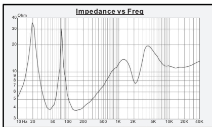
PH-1502阻抗曲线
